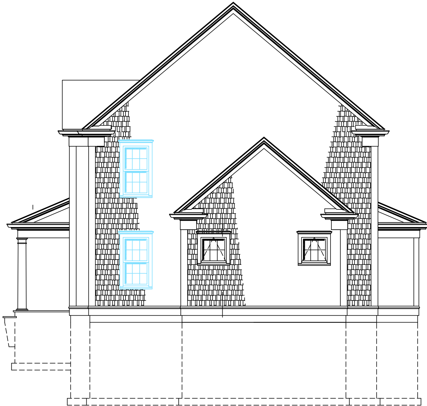
RIGHT ELEVATION
